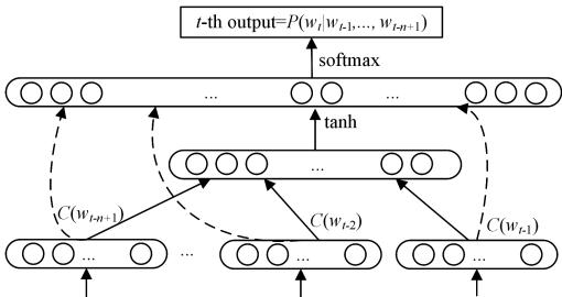
图 1 NNLM 模型的结构 Fig. 1 Structure of NNLM model
