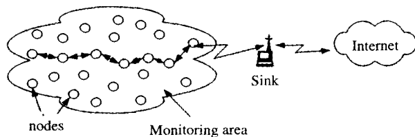
图 1 传感器网络体系结构
