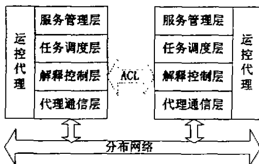
图 3 CIMS 应用集成平台代理单元结构模型
