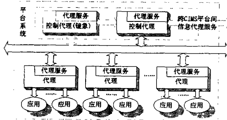
图 2 CIMS 应用集成平台代理整体结构模型
