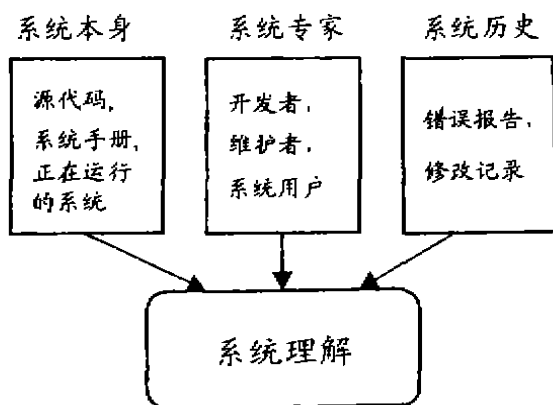
图 5 系统理解的生成
