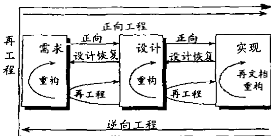
图 1 再工程的定义
