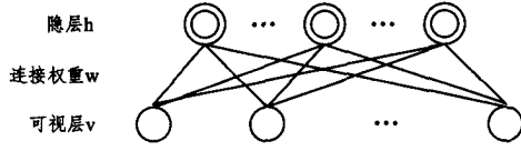
图 2 RBM 模型
