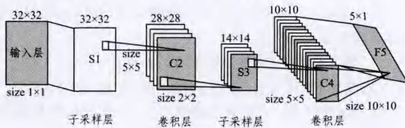
图3 CNN模型
