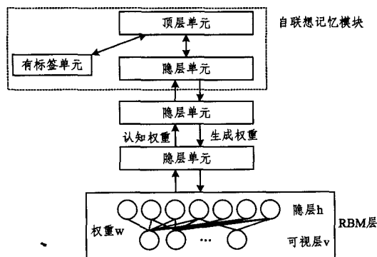
图 1 DBN 模型
