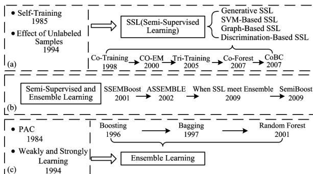
图2 半监督集成学习发展过程
