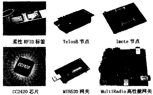
图 4 物联网相关设备和器件
