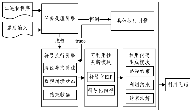
图 7 原型系统 R2dlAEG 的框架图
