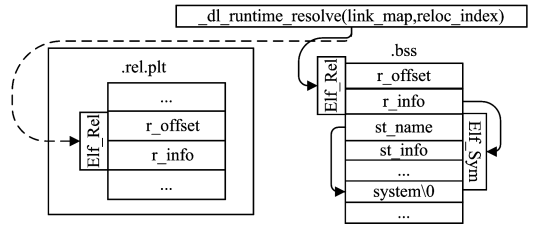
图 2 Return-to-dl-resolve 利用流程图 [6]
