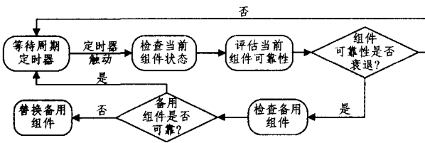
图1 分布式系统中的组件监控替换机制
