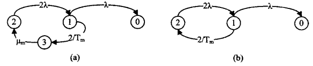
图2 基于监控的冗余组件状态变化模型
