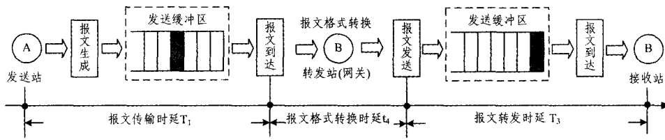
图 8 两点之间通过转发站进行报文传输
