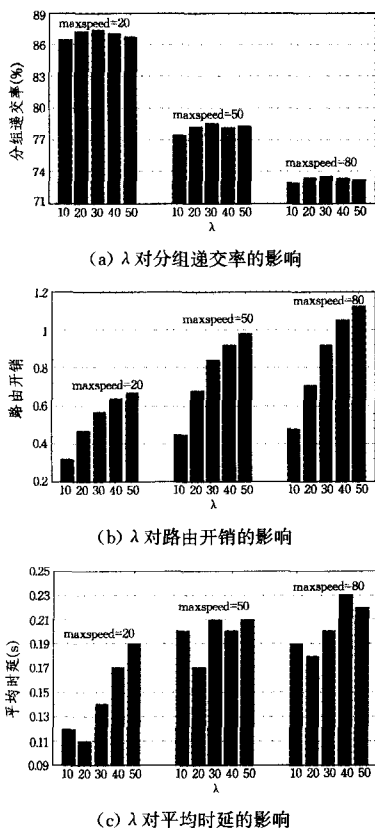
图 4 不同移动速度时调整因子 \lambda 对 GA-ROC 性能的影响
