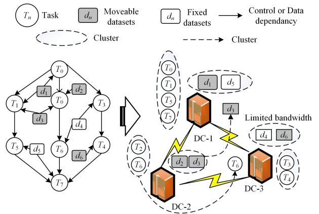
图 3 跨数据中心的任务间通信 [37]
