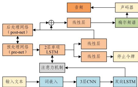
图 1 Tacotron2 模型结构
