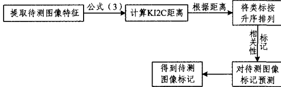
图 1 本文方法对待测图像分类的流程
