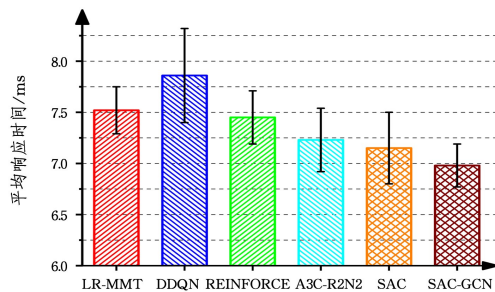
图 9 6 种调度算法下的平均响应时间对比
