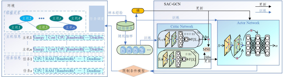
图4 基于 SAC-GCN 模型的架构图
