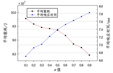
图 5 参数灵敏度分析
