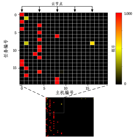
图 6 SAC-GCN 任务偏好图
