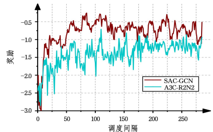
图 7 SAC-GCN 与 A3C-R2N2 的奖励对比
