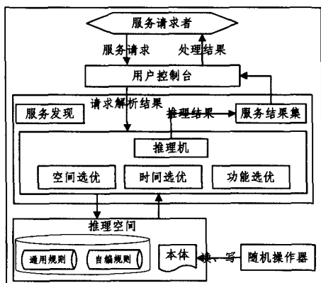
图 4 系统体系结构
