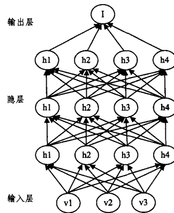
图 2 含多个隐层的深度学习示意图
