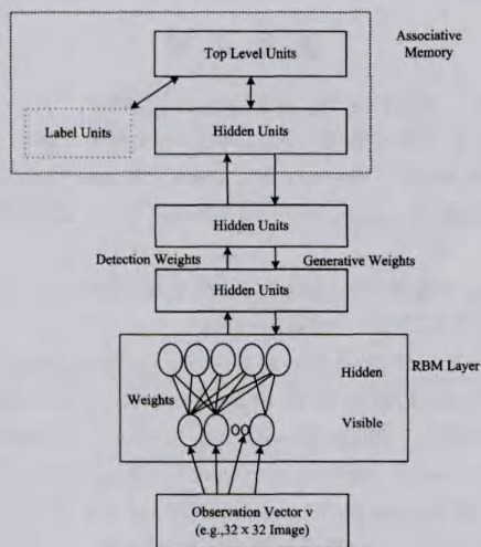
图5 DBN结构
