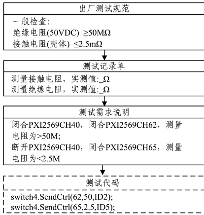
图2 机载设备测试需求开发过程
