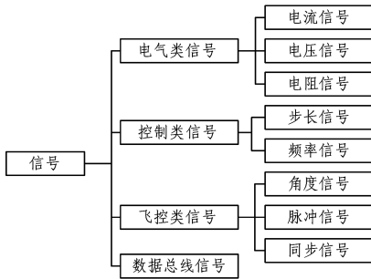
图3 信号分类
