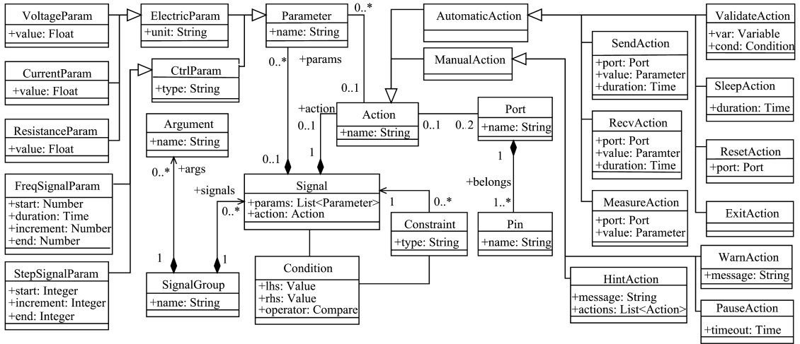
图 6 信号元模型
