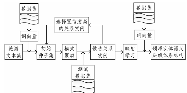
图1 领域实体上下位关系的原理框图
