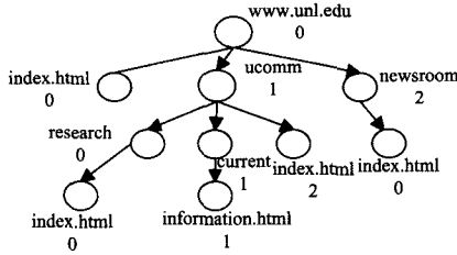
图2 截取某 Web 应用目录树一部分
