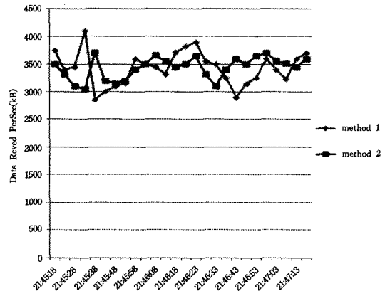
图 4 两种方法对应的 Web 应用吞吐量对比图
