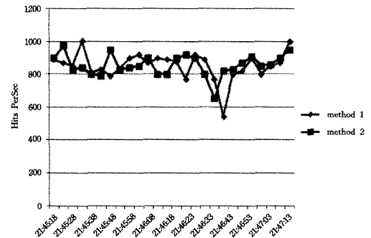
图 5 两种方法对应的 Web 应用 httphits 对比图
