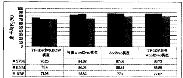
图 6 4 种文档向量分类效果比较
