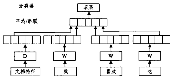
图3 doc2vec 预测模型
