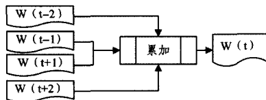
图1 CBOW 模型
