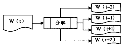
图2 Skip-gram 模型
