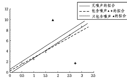
图8 最小二乘法拟合包含噪声数据的效果图
