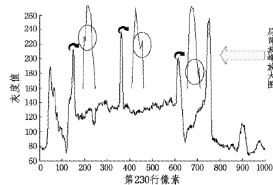
图 5 图 4(a)的第 230 行像素的灰度变化图
