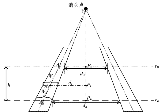
图 11 车道线“位置-宽度”示意图
