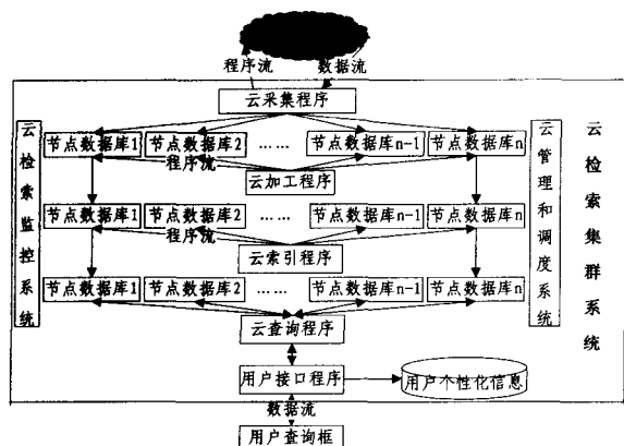
图1 云检索系统架构
