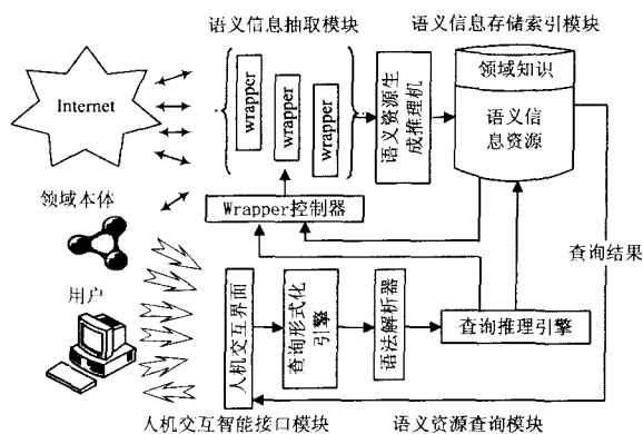
图 1 语义 Web 搜索引擎体系结构
