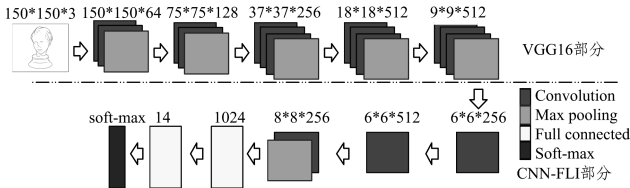
图 5 网络结构图
