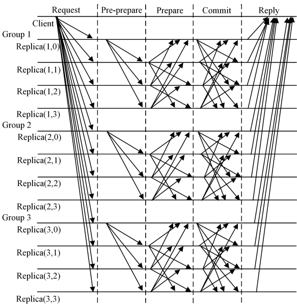
图 4 GPBFT 算法的过程 Fig. 4 Process of GPBFT algorithm
