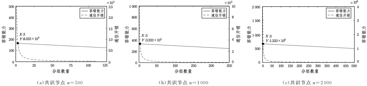
图 7 容错能力与通信开销的关系
