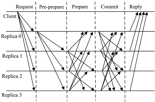
图 3 PBFT 算法的过程 Fig. 3 Process of PBFT algorithm
