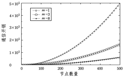
图 6 不同分组下的通信开销对比
