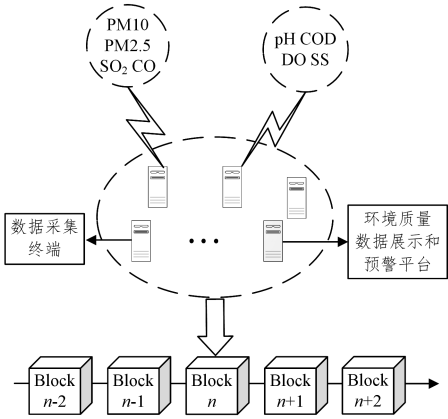
图 1 环境监测区块链方案
