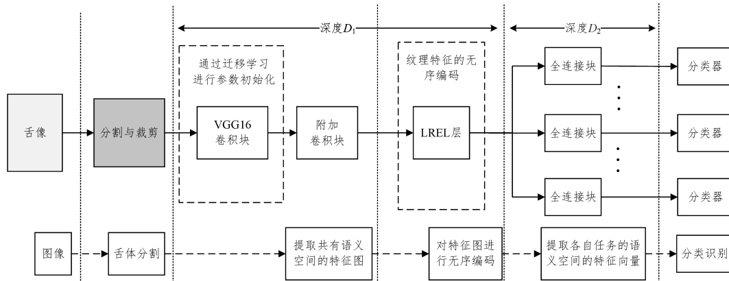
图 5 纹理特征识别模型的基本架构
