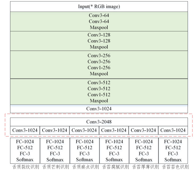
图 14 未使用 LREL 的纹理特征识别模型
