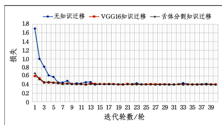
图 11 舌象几何特征分析模型的损失函数变化曲线图
