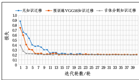
图 15 舌象纹理特征分析模型的损失函数变化曲线图
