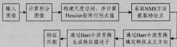
图 1 SURF 算法流程
