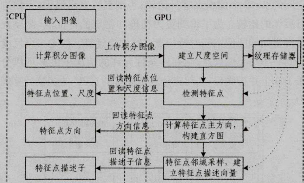
图 3 SURF 算法 CUDA 并行化实现流程图
