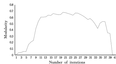
图 1 模块度 Q 的变化
