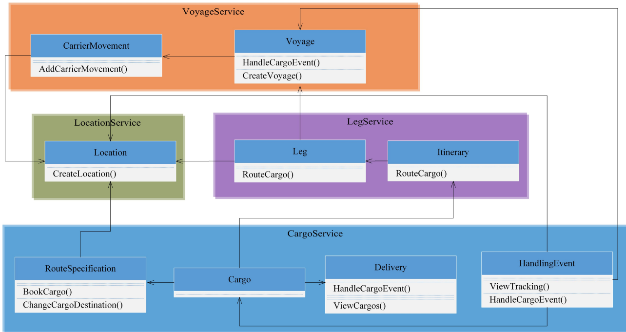
图 2 CTS 的划分结果
