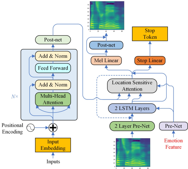
图 4 本文提出的模型架构
