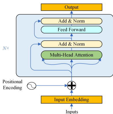
图 3 BERT 架构
