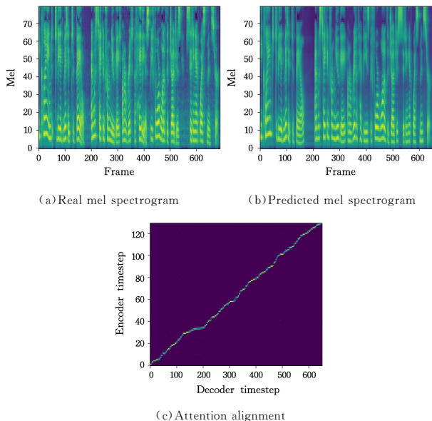
图 5 特征预测
