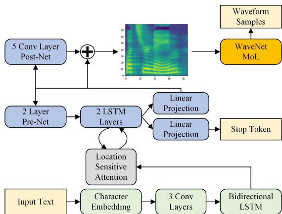
图 2 Tacotron2 架构
