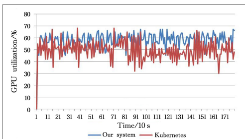
图 3 GPU 利用率对比情况
