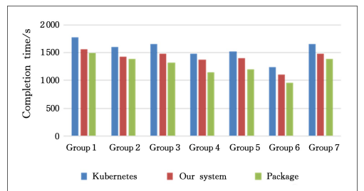
图 5 任务完成总时间对比
