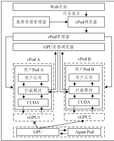
图1 GPU共享调度系统架构图
