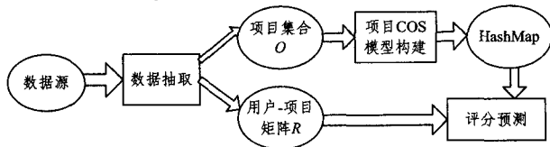
图1 对象耦合相似度下的项目推荐算法框架
