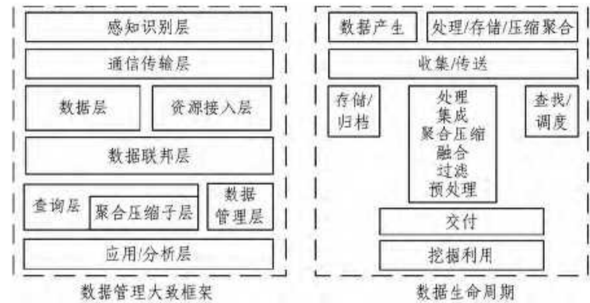
图1 数据管理框架各个堆叠层与数据生命周期的相互映射 1)
