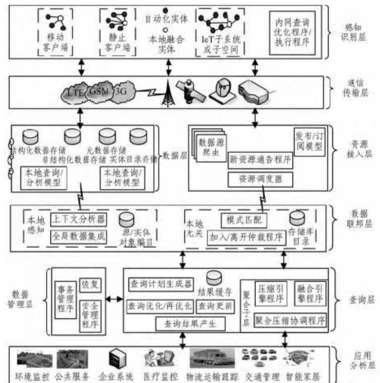
图2 数据管理框架体系结构
