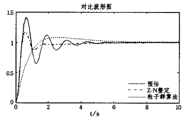
图 9 仿真对比图
