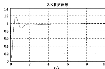
图 5 仿真图
