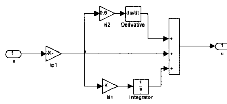
图 4 PID 方块图
