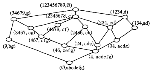
图1 表1的概念格的Hasse图表示
