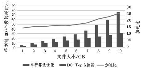
图 9 DC-Top-k 算法与串行算法的性能对比
