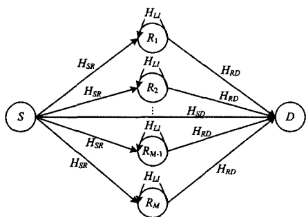
图 1 协作通信全双工中继系统模型
