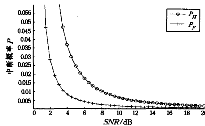
图 4 \pi_{LI_{\min}} = 0.1\text{dB} 时全双工和半双工自适应算法中断概率比较
