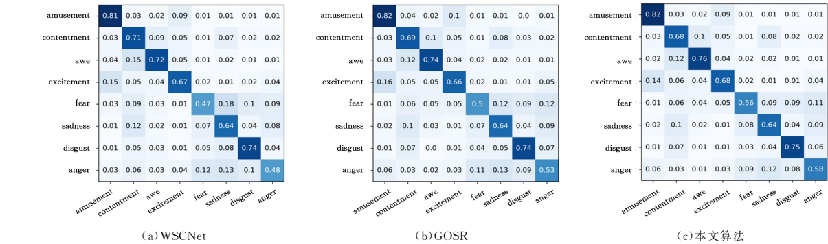
图 5 本文算法和最先进算法在 FI-8 数据集上的分类混淆矩阵
