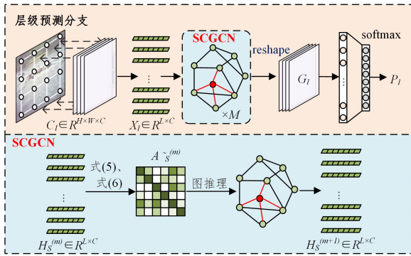
图 3 SCGCN 和层级预测分支
