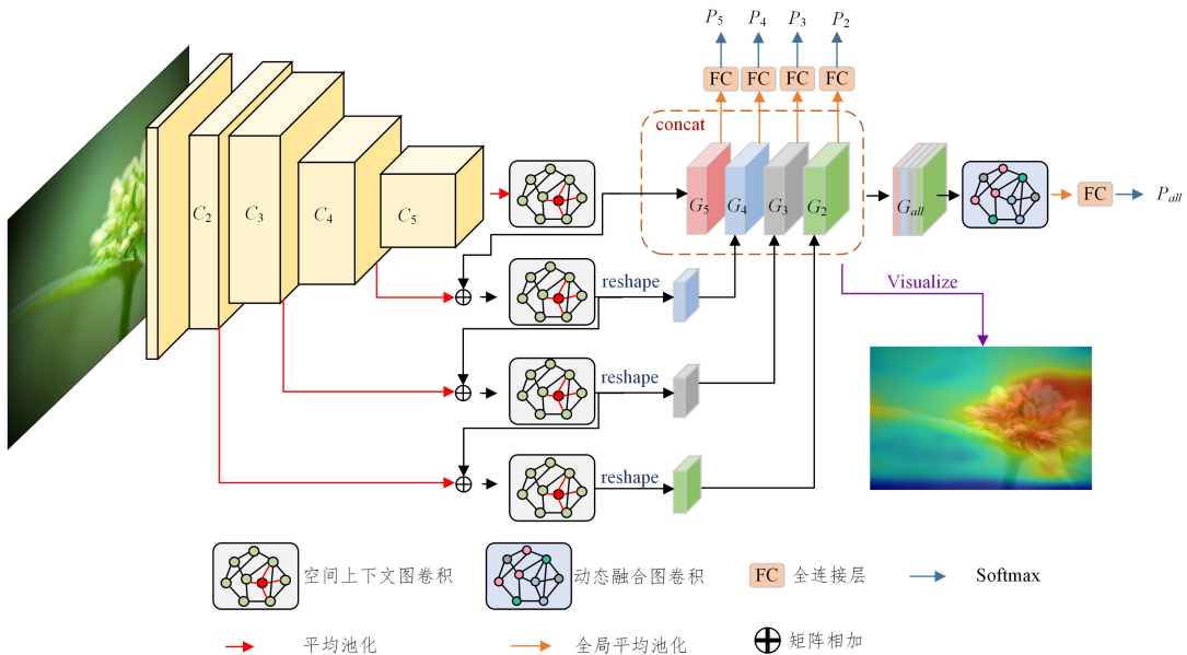
图 2 图像情感分类的层次图卷积网络模型框架
