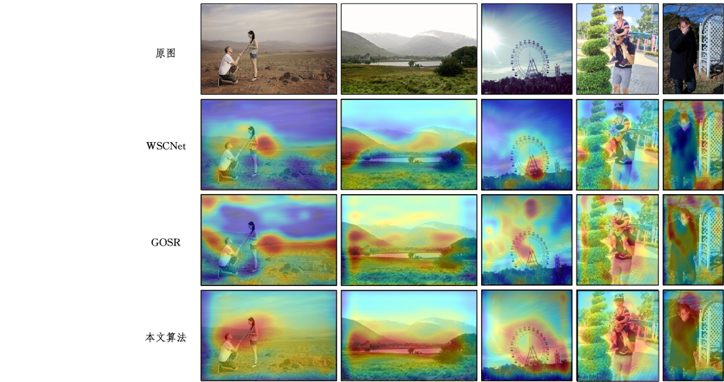
图 6 不同算法的情感感知区域对比
