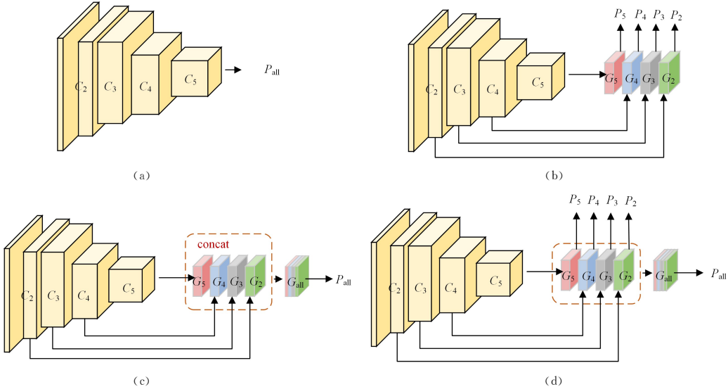
图 7 4 种情感分类架构 Fig. 7 Four sentiment classification architectures
