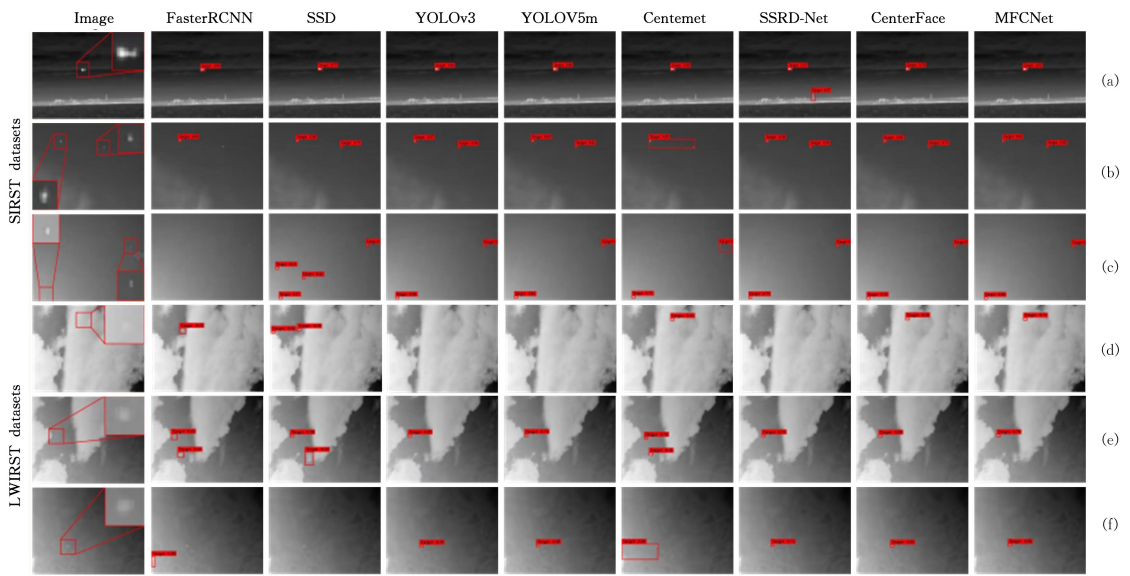
图 5 各算法的检测效果图 Fig.5 Detection effect of each algorithm
