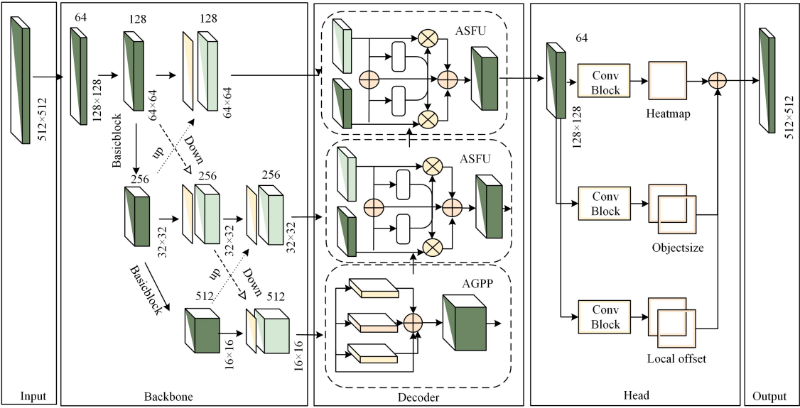
图 1 MFCNet 模型整体结构图 Fig. 1 Overall structure of MFCNet model
