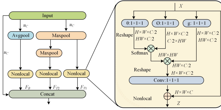
图3 AGPP 结构图
