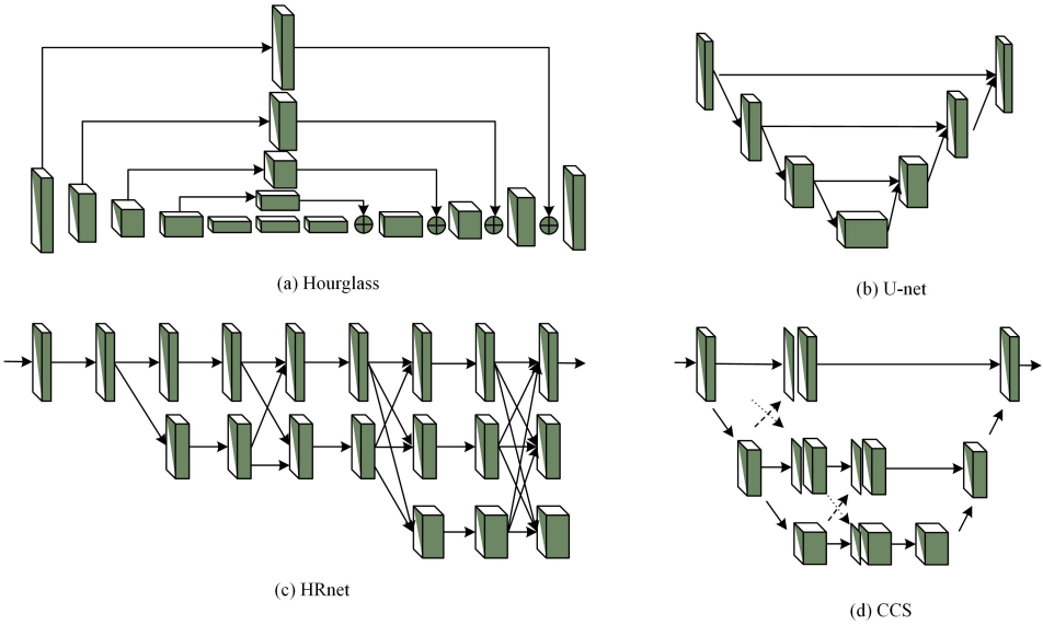
图 2 主干网络结构对比 Fig. 2 Comparison of backbone network structure
